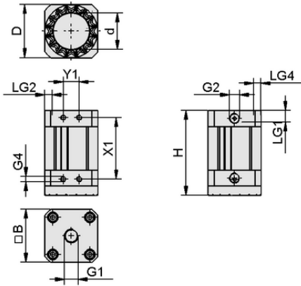
Tasarım verileri SGM 30 G1/8-IG
