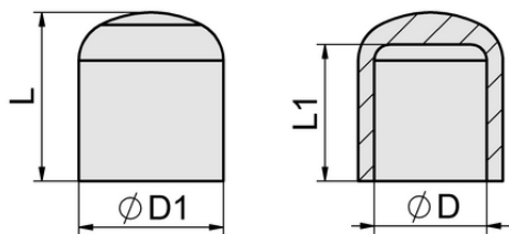
デザインデータ KAPP 7x10.5 SSCB
