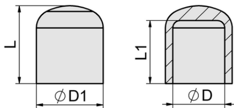
Konstruktionsdaten KAPP 7x10.5 SSCB
