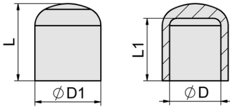
Tasarım verileri KAPP 7x10.5 SSCB
