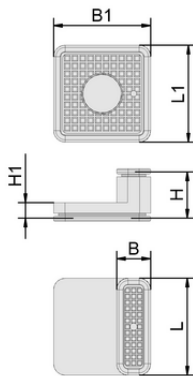
Datos de diseño ISBL-HD 80x28x38
