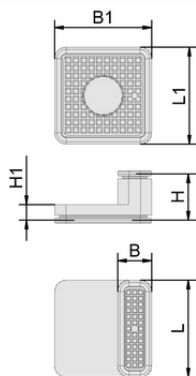
デザインデータ ISBL-HD 80x28x38
