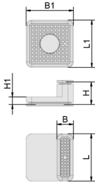
Tasarım verileri ISBL-HD 80x28x38
