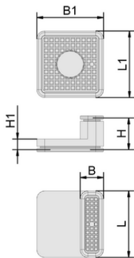
Datos de diseño ISBL-HD 80x40x38
