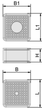
Tasarım verileri ISBL-HD 80x80x38
