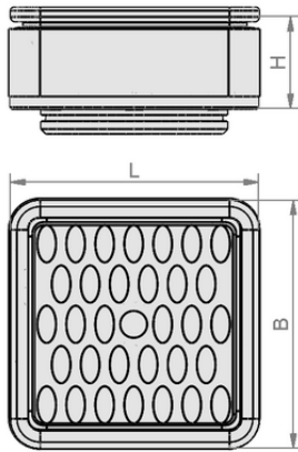
Tasarım verileri ISCUP Cup 4 100x100x30 TV
