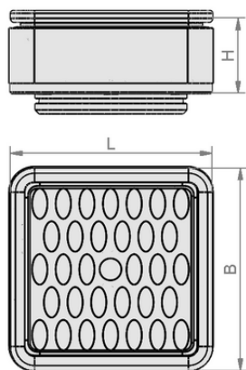
デザインデータ ISCUP Cup 4 100x100x30 TV
