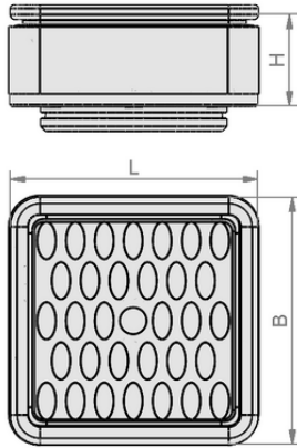
Tasarım verileri ISCUP Cup 4 100x100x30
