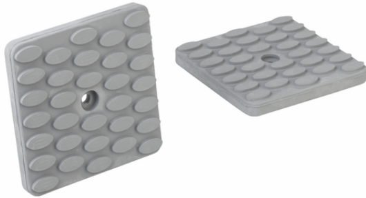
ISRPL 86x86x8.7 NBR-55 d5
