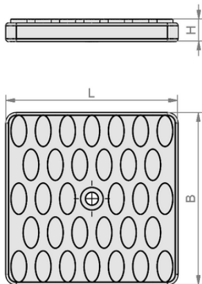
デザインデータ ISRPL 86x86x8.7 NBR-55 d5
