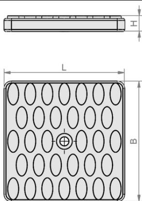
Конструктивные данные ISRPL 86x86x8.7 NBR-55 d5
