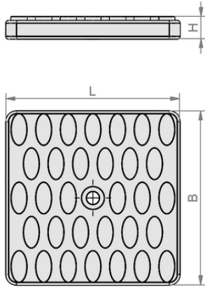
Tasarım verileri ISRPL 86x86x8.7 NBR-55 d5
