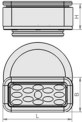
Tasarım verileri ISCUP Cup 2 80x40x30 TV
