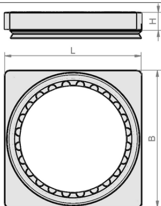
Datos de diseño AP-R-160x160x16-50x50
