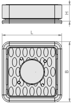
Tasarım verileri ISMB 80x80x26
