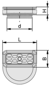
Tasarım verileri ISCUP Cup 2 80x40x16
