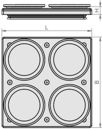
Tasarım verileri ISQB-R 175x175x15 30/50
