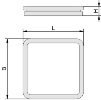
Tasarım verileri ISDR 167x167x9.3 NBR-55
