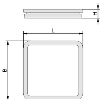
Données de construction ISDR 167x167x9.3 NBR-55
