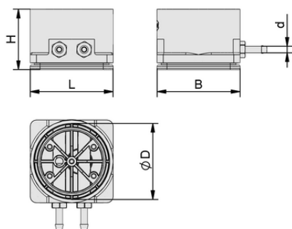
デザインデータ ISMB-G 80x80x70
