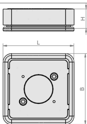
Datos de diseño ISMB-T 80x80x22
