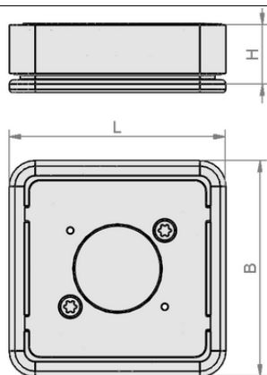
デザインデータ ISMB-T 80x80x22
