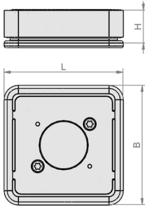
Tasarım verileri ISMB-T 80x80x22
