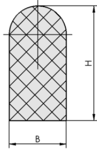
Tasarım verileri DI-PROF 4x10 MOS EPDM HR
