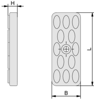
Tasarım verileri ISRPL 66x66x8.5
