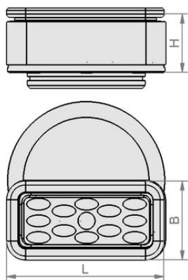
デザインデータ ISCUP Cup 3 80x28x30
