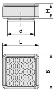
デザインデータ ISCUP Cup 1 80x80x30
