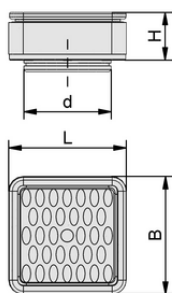
Datos de diseño ISCUP Cup 1 80x80x30
