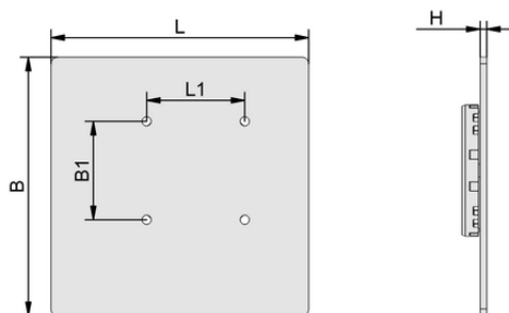
デザインデータ ISAP-S6 200x200x30
