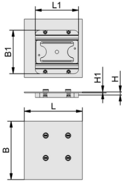
Tasarım verileri ISAP-S4 195x195x11
