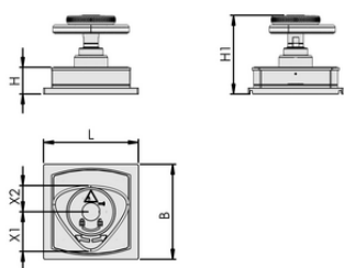
デザインデータ VCMC-R-QUICK 160x160x45 30/40/50
