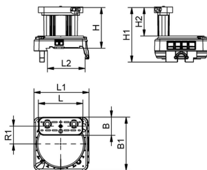
Dati di costruzione VCBL-S6 120x50x50 S-360-15 TV
