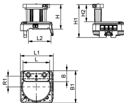
Données de construction VCBL-S6 130x30x75 S-360-15 TV
