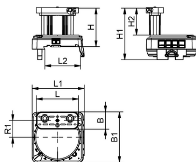
Dati di costruzione VCBL-S6 130x30x75 S-360-15 TV
