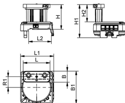
Données de construction VCBL-S6 120x50x75 S-360-15 TV
