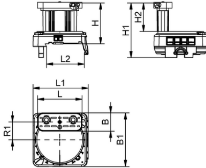
Tasarım verileri VCBL-S6 130x30x110 S-360-15 TV
