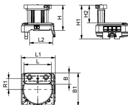
Dati di costruzione VCBL-S6 125x75x110 S-360-15 TV+ME
