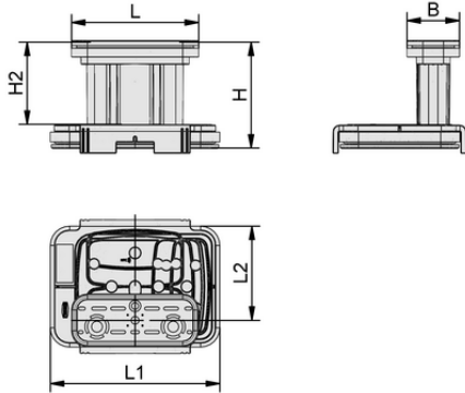
Tasarım verileri VCBL-K2-PRO 120x50x100 L
