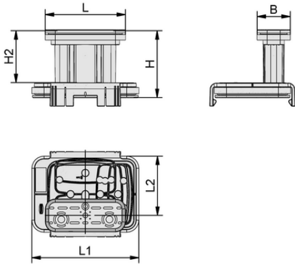
Tasarım verileri VCBL-K1-PRO 130x30x100 L
