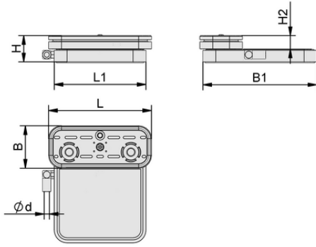
Tasarım verileri VCBL-G-K1 120x50x30
