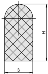
Конструктивные данные DR 178.3/170.25x6 MOS NK-20
