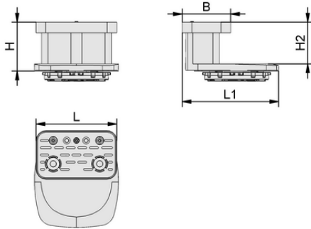
Tasarım verileri VCBL-B 120x50x74 TV
