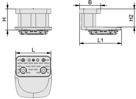
Tasarım verileri VCBL-B 125x75x74 TV
