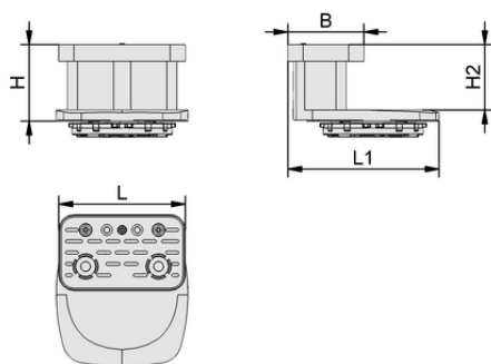
Datos de diseño VCBL-B 125x75x74 TV
