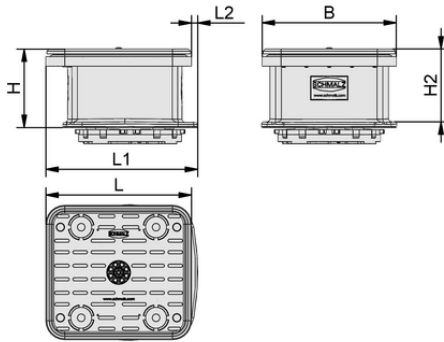
Tasarım verileri VCBL-B 140x130x74 TV
