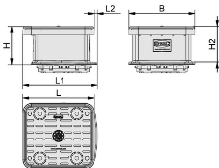
Конструктивные данные VCBL-B 140x130x74 TV
