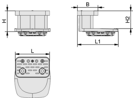
Datos de diseño VCBL-B 120x50x48 TV
